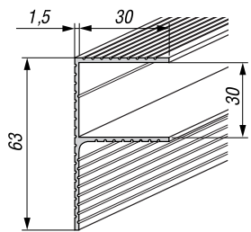
для обрамления шовной доски
