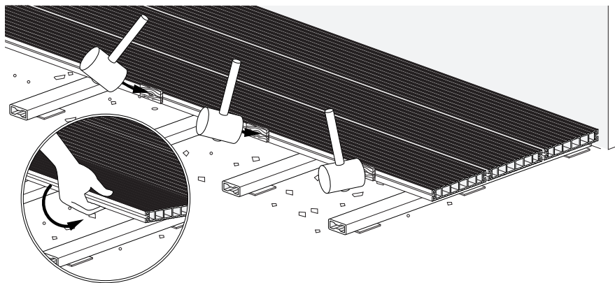
Рис.12 Дальнейшая укладка шовной террасной доски DeckRa
