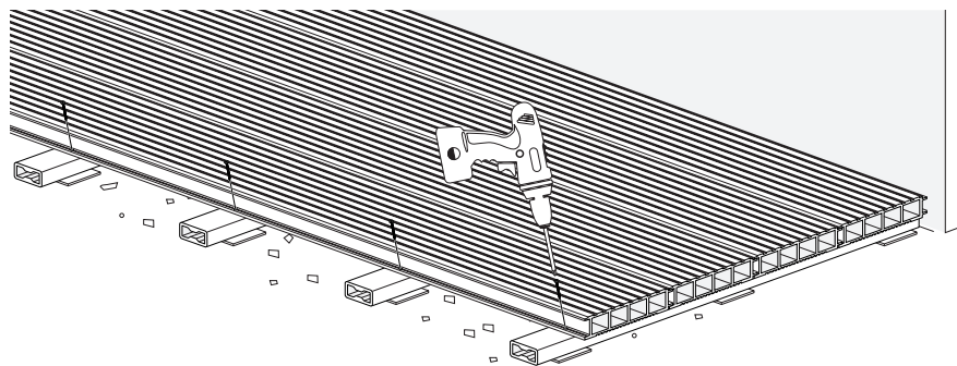
Рис.17 Дальнейшая укладка бесшовной террасной доски DeckRa
