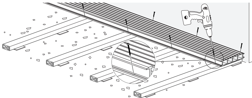
Рис.14 Начало укладки бесшовной террасной доски DeckRa
