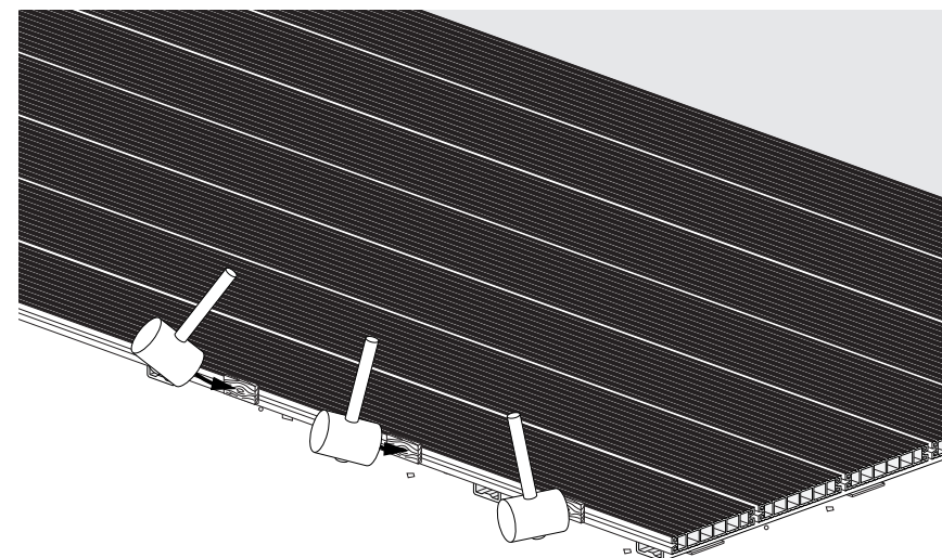
Рис.13 Окончание укладки шовной террасной доски DeckRa
