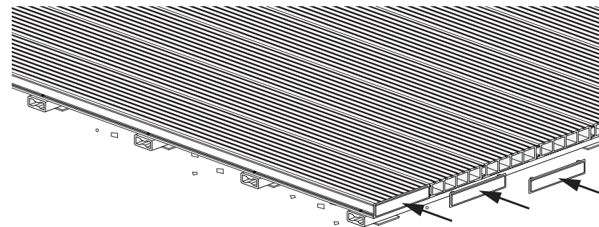
Рис.18 Окончание укладки бесшовной террасной доски DeckRa
