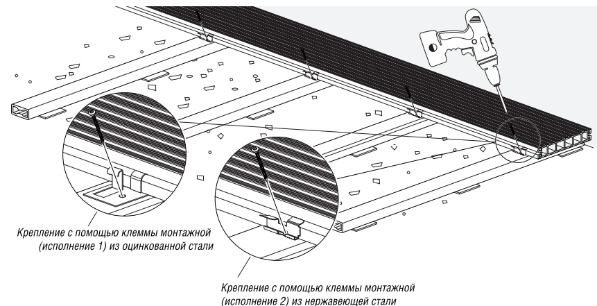
Рис.11 Начало укладки шовной террасной доски DeckRa
