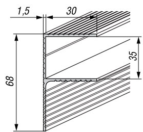
для обрамления бесшовной доски
