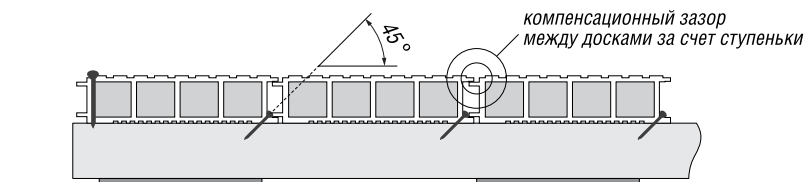
Рис.15 Крепление начального и последующих профилей DeckRa
